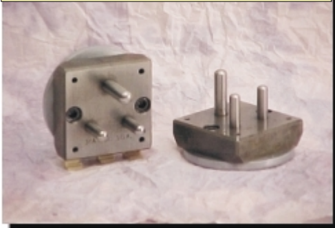
Max. / Min. GO Gauges for 16A Sockets
