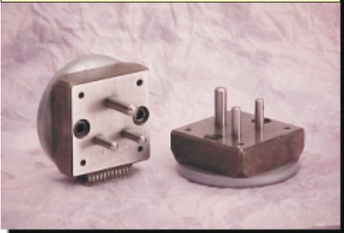
Max. / Min. GO Gauges for 6A Sockets
